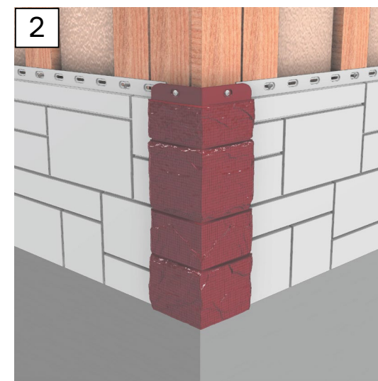
Рис. 22 Монтаж первого ряда панелей
