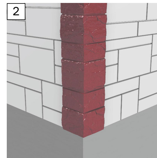
Рис. 23 Монтаж последующих рядов панелей
