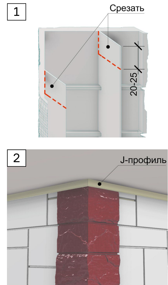
Рис. 27 Примыкание внешнего угла Döcke к карнизному свесу.
