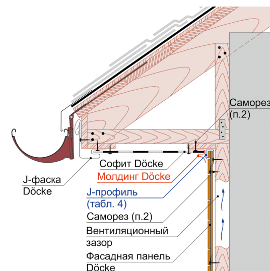
Рис. 25 Примыкание фасадных панелей Döcke к карнизному свесу.
