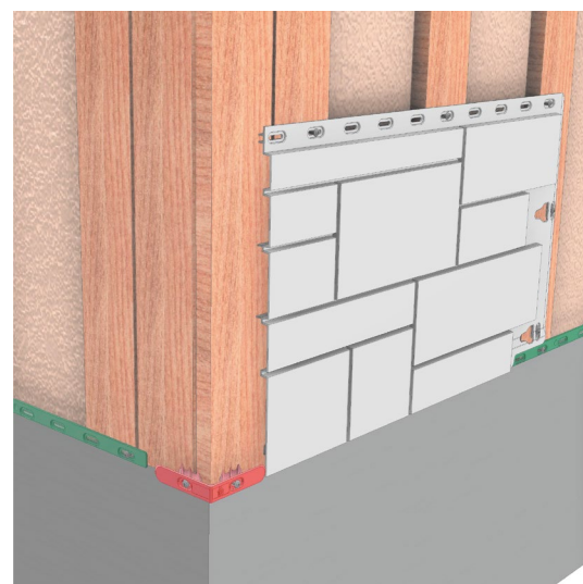
Рис. 21 Монтаж первой панели
