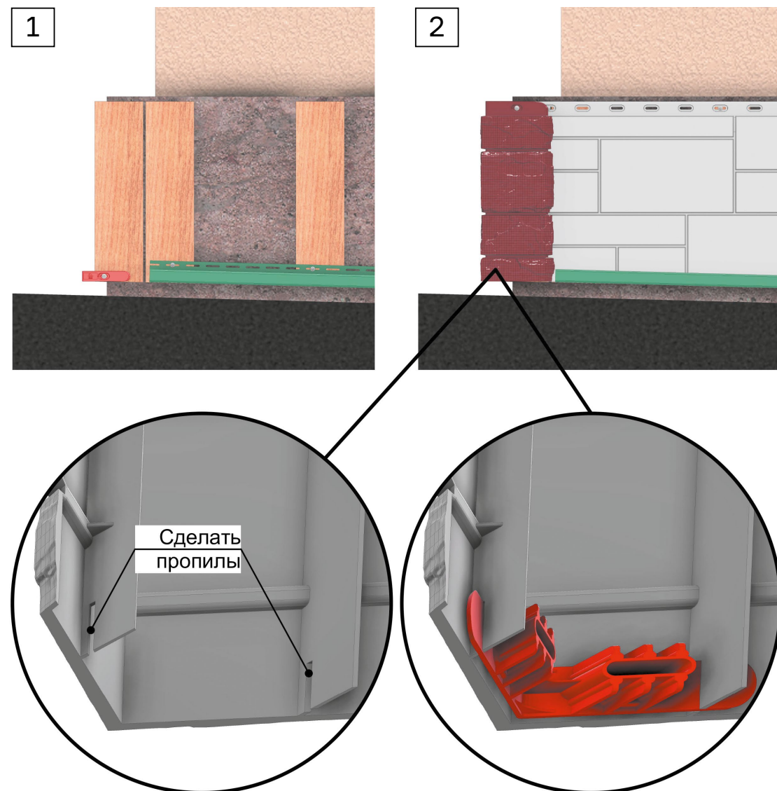
Рис. 24 Отделка цоколя с перепадом высоты
