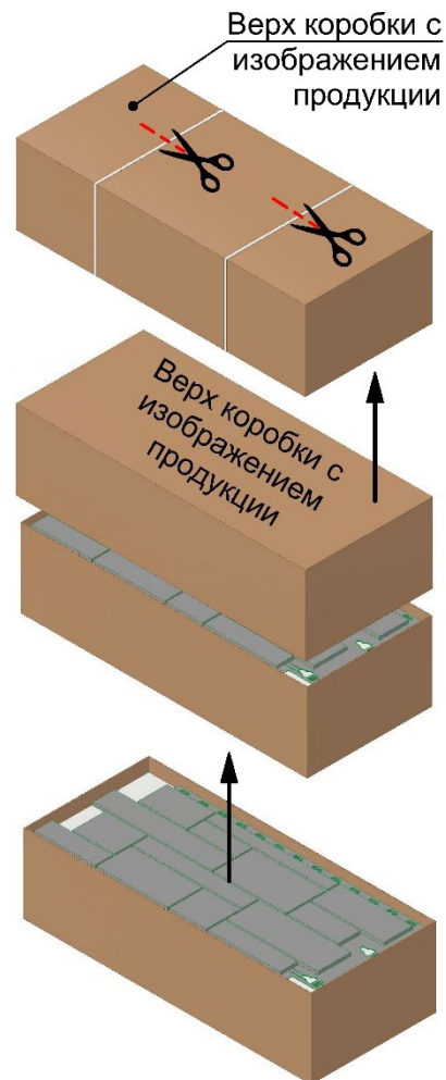
Рис. 20 Схема распаковки
